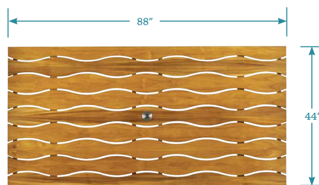
3401-876TT Très Chic Rectangular Dining Table Top 88W x 44D x 1.75H in.
